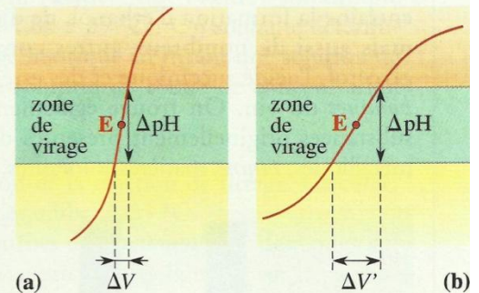
Doc. 14 (a) \Delta \text{pH} est brusque : le titrage est précis ; (b) \Delta \text{pH} est plus étalé : le titrage est imprécis, \Delta V' > \Delta V .
